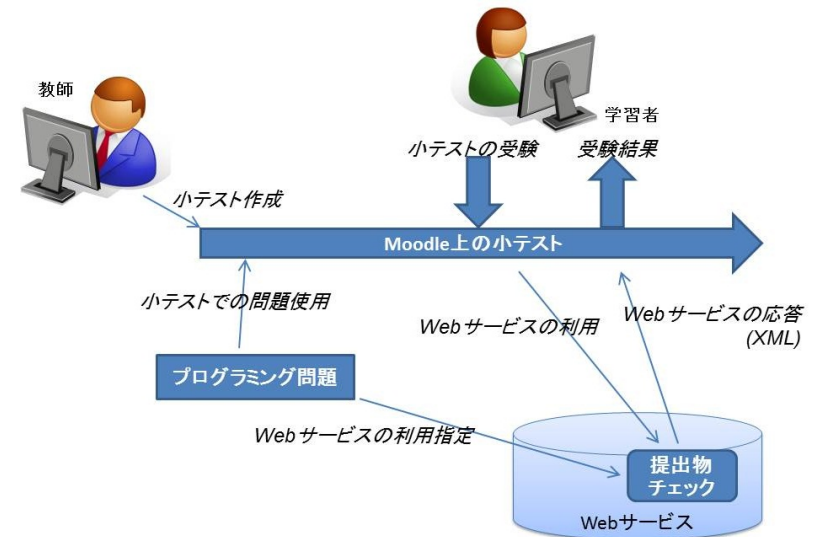
図 3 利用の流れ Fig. 3 Service Flow
