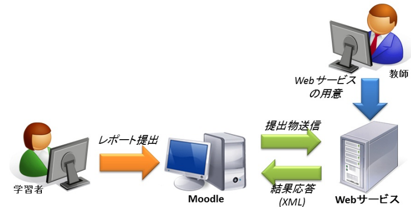
図 2 システム構成 Fig.2 System Architecture
