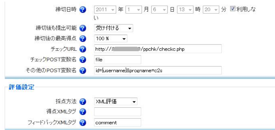
図 4 プログラミング問題の設定画面 (締切および評価設定部分) Fig. 4 Screenshot of Configuration for Programing Question(Deadline and Scoring)
