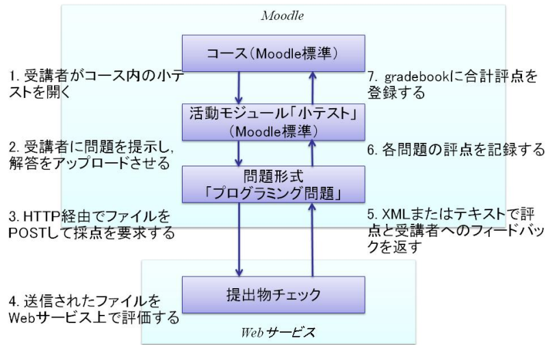
図 5 小テスト全体の処理の流れ Fig. 5 Processing Flow of Whole Quiz
