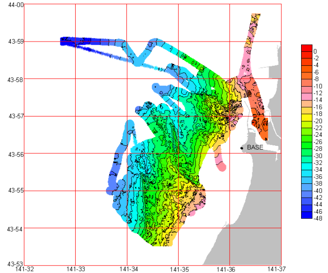
図 2 三次元海底地形図 (コンタ図)
